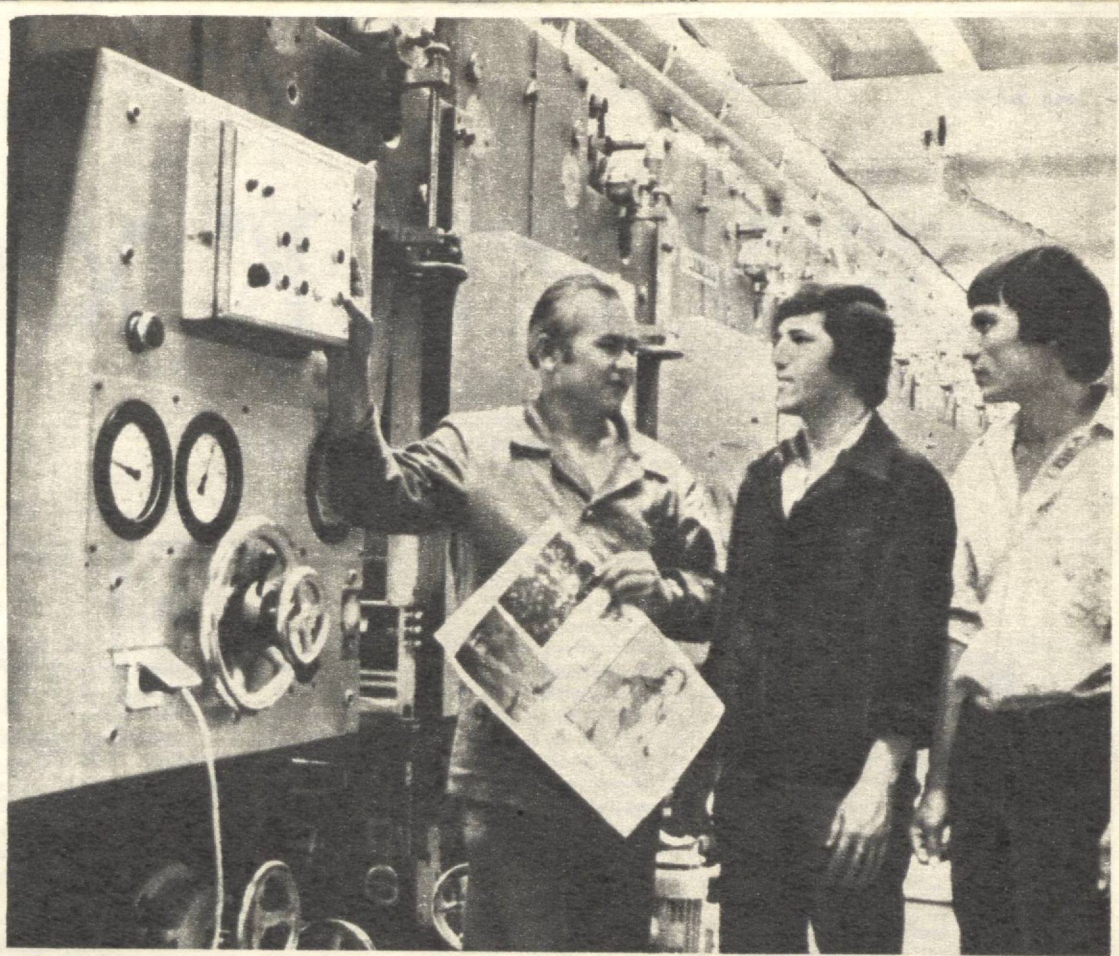
Бир йўла саккиз хил бўёқ бериш имкониятига эга бўлган мана бу машина ҳам Ботиқ цехида муттасил ишлаб турибди. Суратда: мастер Ҳошим Дадашев, печатник Абдулла Назиров ва Аҳаджон Алиевлар янги зарварақларни босиб чиқаришга ҳозирлик кўраётирлар.
