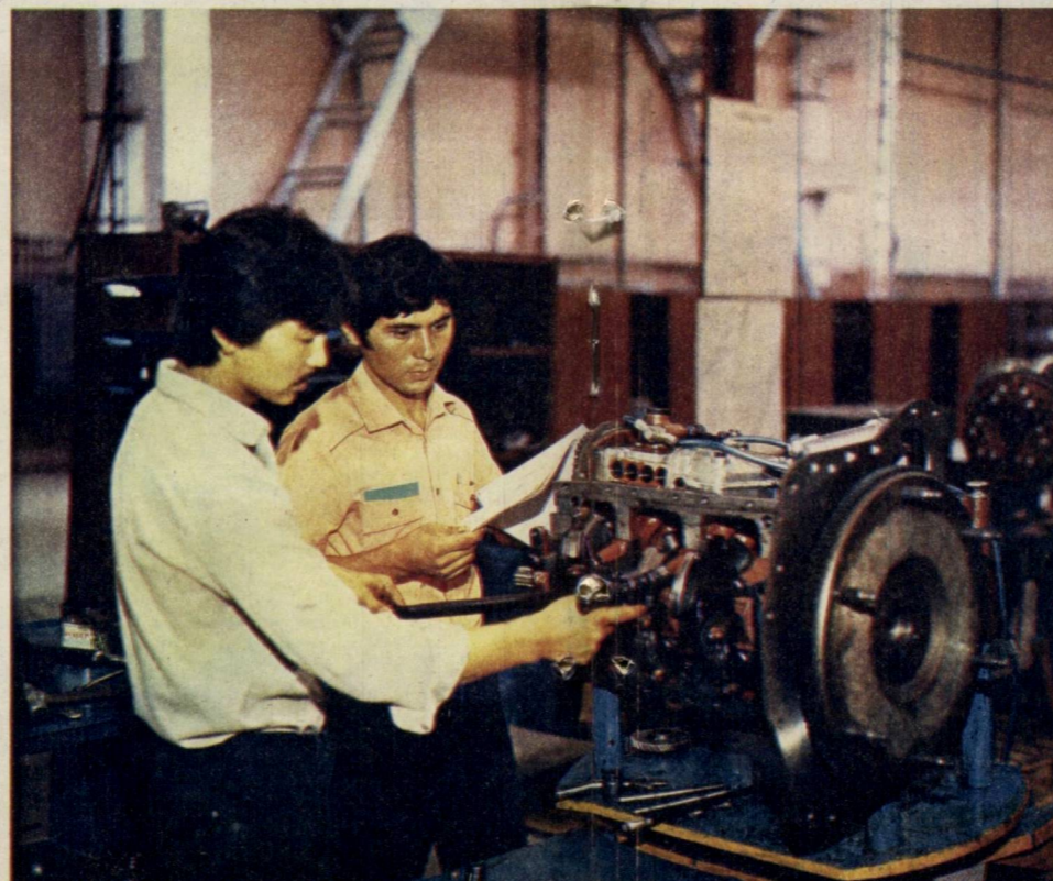
Ийгувчи-слесарь Б. Сулаймонов ва мастер А. Турсунов дастлабки моторларни йиғишда иштирок этмоқдалар.
