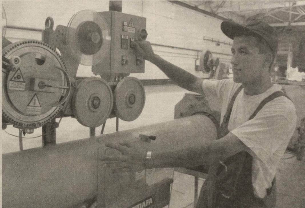
Қарши шаҳридаги «Қарштермопласт» заводи Германия технологияси асосида жиҳозланган. Айти пайта ушбу корхонада йигирма бешдан зиёд турли хил ўлчамдаги полиэтилен қувурлари ишлаб чиқарилиб, республикамиз вилоятларида жўнатилмоқда. СУРАТДА: оператор Бехзод Орзиев.
