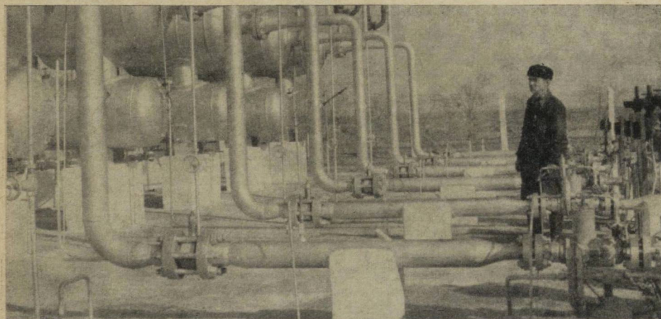
Қашқадарёдаги «Муборак» конининг ўзигина йилига 15 миллиард кубометр мовий ёнилғи беради. Суратда: Октябрь 50 йиллиги номидаги коннинг газ йиғиш пунктларидан бири.
