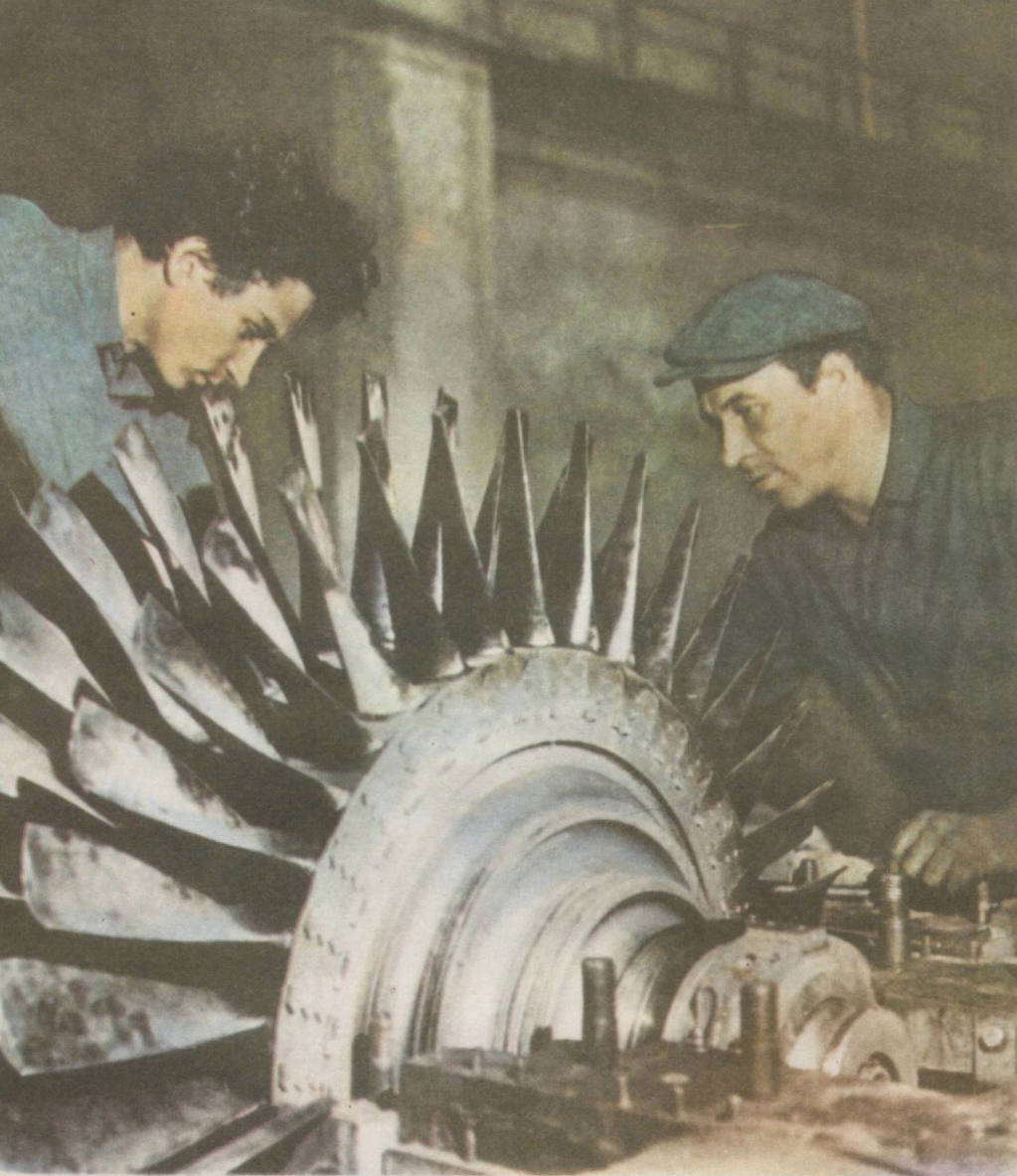
Урта Осиё — Марказ газопроводи Қўнғирот компрессор станциясида слесарлардан В. Свечников ва Н. Кмовин турбина монтаж қилмоқда.
