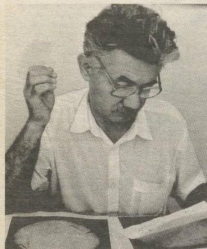
Куёшшунос олим Исроил Сатторов АФР-3 хромосфор телескопи орқали олинган суратларни кўздан кечирмоқда.
