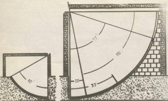
Улуғбек расадхонасининг қурилмаси билан Тихо Брагенин «Ураниборг» расадхонаси қурилмалари ўртасида кузатиш жараёнида фарқ бўлган. Суратда ушбу фарқ тасвирланган [мақолада бу ҳақда батафсил маълумот берилган].
