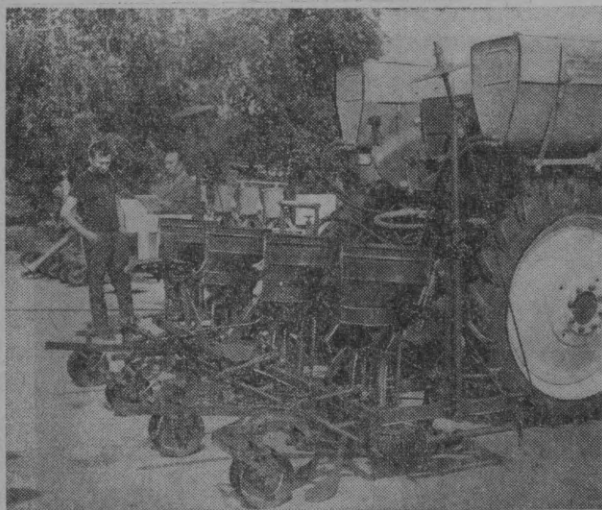
Шу кунларда Ўзбекистон халқ хўжалиги ютуқлари кўрғазмасига кўйилган ва «Ўзбексельмаш» заводининг машинасозлари томонидан тайёрланган кенг қаторли янги «СЧХ-4А-1» маркали чигит экиш сеялкаси томоабдиллар диққатини ўзига тортмоқда.
