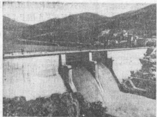
Югославия. Дубровника яқинидаги Трешбишница дарёсига «Дуброник» электрстанцияси қурилмоқда...
