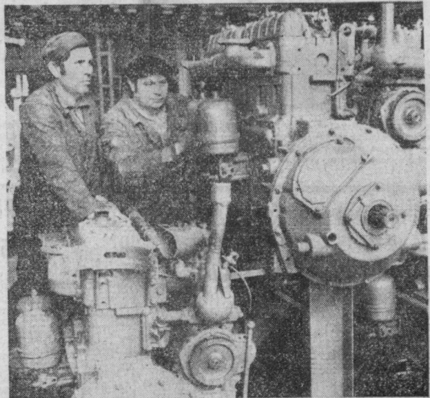
«Госкомсельхозтехника»нинг Қўйли қадаги тақриба-ремонт механика за-води мотор цехи коллективи бу йил 7,5 мингта трактор дингательини қай-та тиклаб берди. Цехда дингательларни тез ва соз ремонтдан чиқариш учун барча шароитлар яратилди. СУРАТДА: мотор цехининг В. Ко-ловский бошлиқ бригадаси йиғувчи лари соланган дингательларни жуна-тиш учун ҳўзирламоқдалар.
