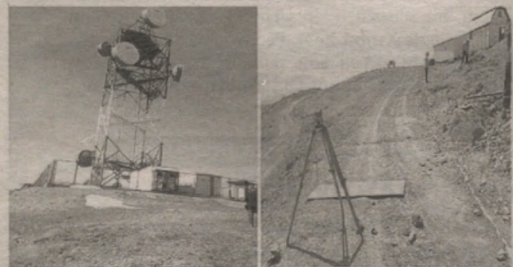
Гибрид қуёш-шамол-дизел электростанциялари қурилишининг бориши
