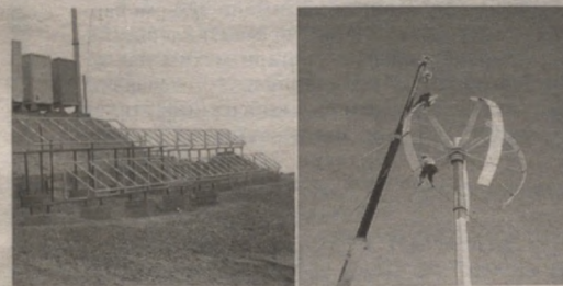
Гибрид қуёш-шамол-дизел электростанциялари қурилишининг бориши
