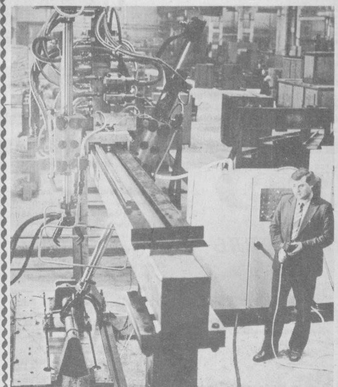
Бошқирдистон АССР. Стерлитамадаги аниқ ҳисобли станоклар заводда программали бошқариладиган робот-манипуляторлар қўллаб ишлаб чиқарилмоқда. Бу ерда ишлаб чиқариладиган роботлар мамлакатимиздаги заводларга жўнатилаётган. Завода ишлаб чиқариладиган робот-манипуляторлар Венгрияда ўтказилади саноат ярмаркасида намоиш этилди. СУРАТДА: робот-манипуляторлар сновдан ўтказилмоқда.
