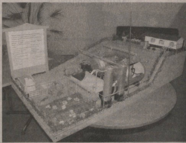
Фермер хўжалиги учун қурилган чорва, парранда ва ўсимлик чикиндиларини қайта ишлаш биогаз қурилмаси макети.
