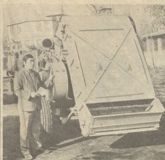
Новый воздухоочиститель марки УПХ-1,5 «Г» запущен в серийное производство «Узбексельмаш». Новый агрегат от предыдущих моделей отличается повышенной производительностью, специальным фильтром для очистки хлопка от пыли и мусора, экологическая чистота и надежность в эксплуатации, что доказали его отличные испытания в хлопковых хозяйствах нашей республики. Воздухоочиститель монтируется с тракторами или приводится в движение электроприводом ЭП-1. В этом году коллектив объединяет изготовит 2.800 штук таких воздухоочистителей.
