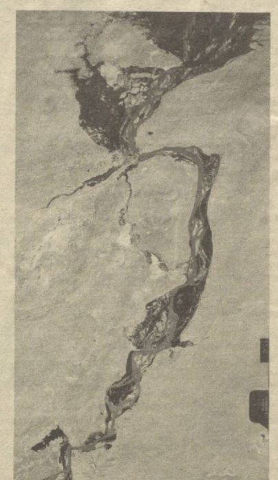
Эти снимки получены из космоса. Арал (снимок слева) почти разделен на две части. Снимок справа сделан до появления на Амударье Тулымского гидроузла. Хорошо видны соленые озера (светлые). На снимке внизу — Каракумский канал. Темные пятна — выход на поверхность в результате инфильтрации подземных вод.
