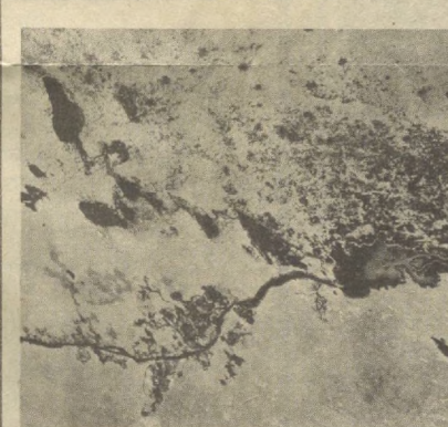
Арал (снимок слева) почти разделен на две части. Снимок справа сделан до появления на Амударье Тулымского гидроузла. Хорошо видны соленые озера (светлые). На снимке внизу — Каракумский канал. Темные пятна — выход на поверхность в результате инфильтрации подземных вод.
