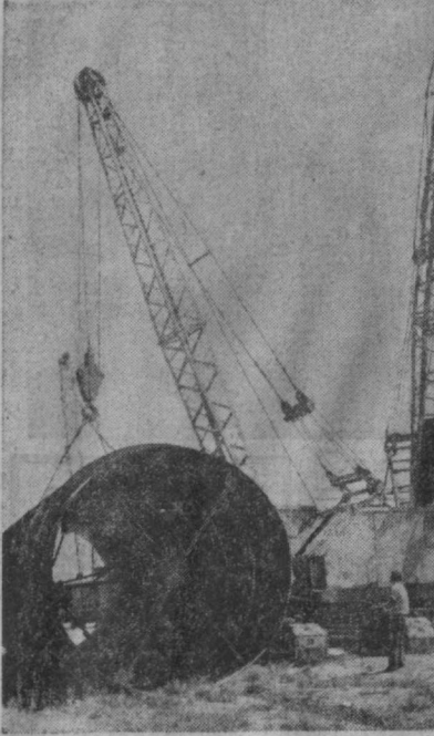
В Днипровской степи создается крупная магистральная ирригационная система, с вводом ее в действие будут подготовлены и посею хлопчатника 175 тысяч гектаров новых земель. На снимке: монтаж водовода ведут рабочие ПМК-2 треста «Ирригация».
