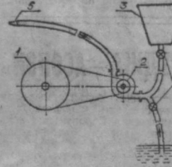
(1) — шкив на валу отбора мощности; (2) — шкив на валу привода насоса; (3) — ем-
