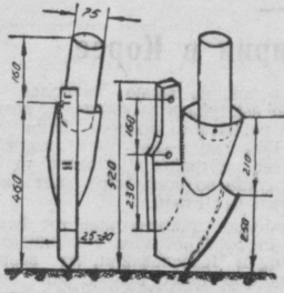
рабочий орган для внесения минеральных удобрений
