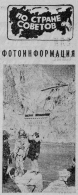
Много хлопот у работников Токтогульской ГЭС, наблюдающих за «поведением» 215-метровой железобетонной «плотины». В ее теле установлено свыше двух с половиной тысяч приборов. Большую помощь эксплуатационникам, ведущим себя «плотина», оказывают водолазы, которых вы видите на снимке.
