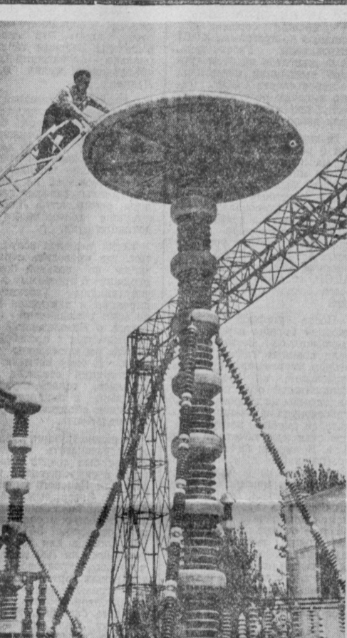
В лаборатории высоких напряжений Научно-исследовательского института энергетик и автоматики ведется работа по испытанию новых мощных изоляторов для линий электропередач. На снимке: подготовка электрических изоляторов к испытаниям.
