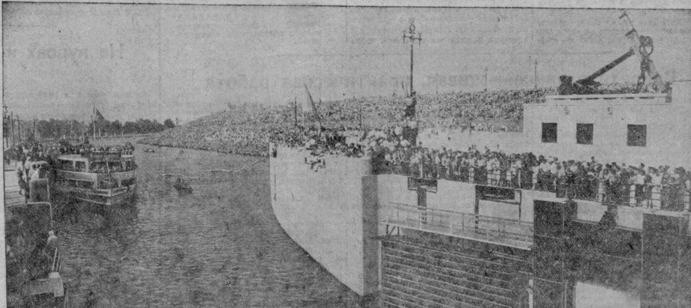
Торжественное открытие Волго-Донского судоходного канала имени В. И. Ленина 27 июля 1952 года. На снимке: теплоход «Иосиф Сталин», открывший pravidelное движение на канале, входит в первый шлюз. На снимке: теплоход «Иосиф Сталин», открывший pravidelное движение на канале, входит в первый шлюз. Фото С. Иропаничного. (Фотохроника ТАСС).
