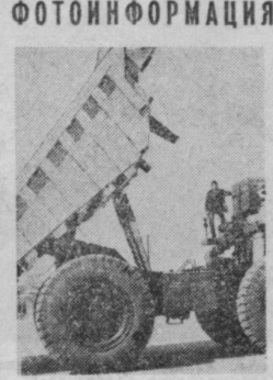
БЕЛОРУССКОЕ объединение по производству большегрузных автомобилей имени 60-летия Великого Октября — одно из крупнейших в стране. Оно выпускает свыше 30 модификаций машин грузоподъемностью от 8 до 180 тонн. На снимке — 75-тонный самосвал БелАЗ-549.
