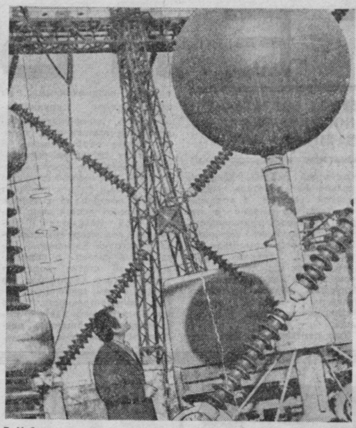
В Узбекском научно-исследовательском институте энергетик и автоматизации Минэнерго СССР проводится большой комплекс работ, связанных с повышением надежности изоляции сверхвысоковольтных линий электропередач. На снимке: идет подготовка к очередному эксперименту на установке в один миллион вольт. (Фотохроника УэТАУ).
