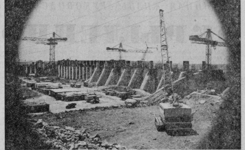
Проектной высоты достигла плотина Тямуюнского гидроузла. Сейчас на строительстве этого самого крупного в Средней Азии гидротехнического сооружения началась предпроектная пора — коллектив треста «Тямуюн-гидрострой» начал подготовку к перекрытию соосеивающей Аму-Дарьи. На снимке: строительство Тямуюнского гидроузла. Фото К. АТАЕВА (УзТАГ).
