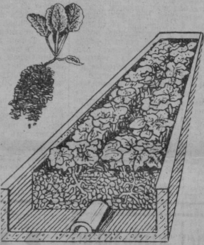
На верхнем рисунке — рассада помидоров, выращенная гидропонным способом в Институте овоще-бахчевых культур и картофеля. В качестве субстрата-среды использовалась рисовая шелуха. Внизу — схема гидропонной установки на гравии. На переднем плане — труба, через которую подается питательная среда и корневая система растений.
