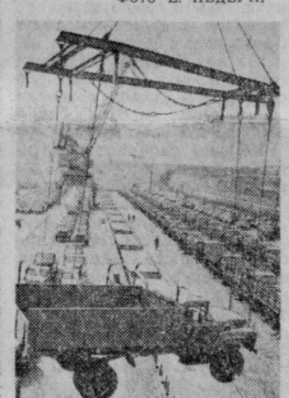
Московский автомобильный завод имени Дзержинского по точному графику отправляет грузовой в сельскохозяйственные районы страны, где идет уборка зерновых. На снимке: на железнодорожной ветке автозавода грузовой машины ставят на платформы для отправки в дальний путь. Фото В. ХУЛАЕВА.
