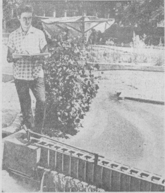
Для строительства гидротехнического сооружения необходимо сделать его модель и провести испытания. Эту работу ведет Институт водных проблем и гидротехники. На снимке: старший техник Эмир Аббас испытывает модель Тюльминского гидроузла на Аму-Дарье.
