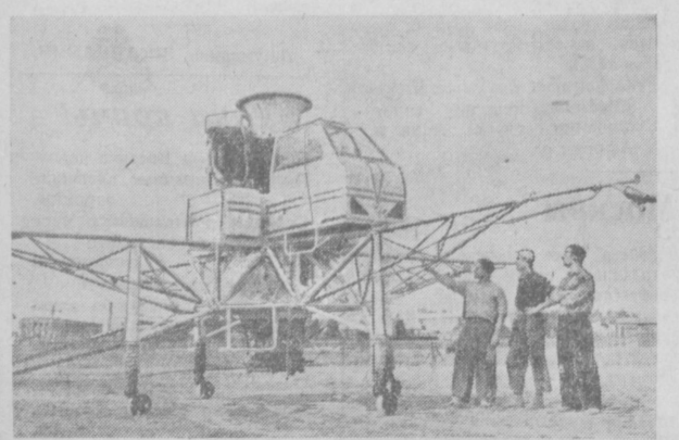
Разработанный конструктором А. Н. Рафаэлянцем турбокомпрессор, так называемый «летающий стол», будет продемонстрирован в полете в День авиации на Ташкентском аэродроме под Москвой. На снимке: турбокомпрессор «летающий стол». Фото В. Третьякова. (Фотохроника ТАСС).
