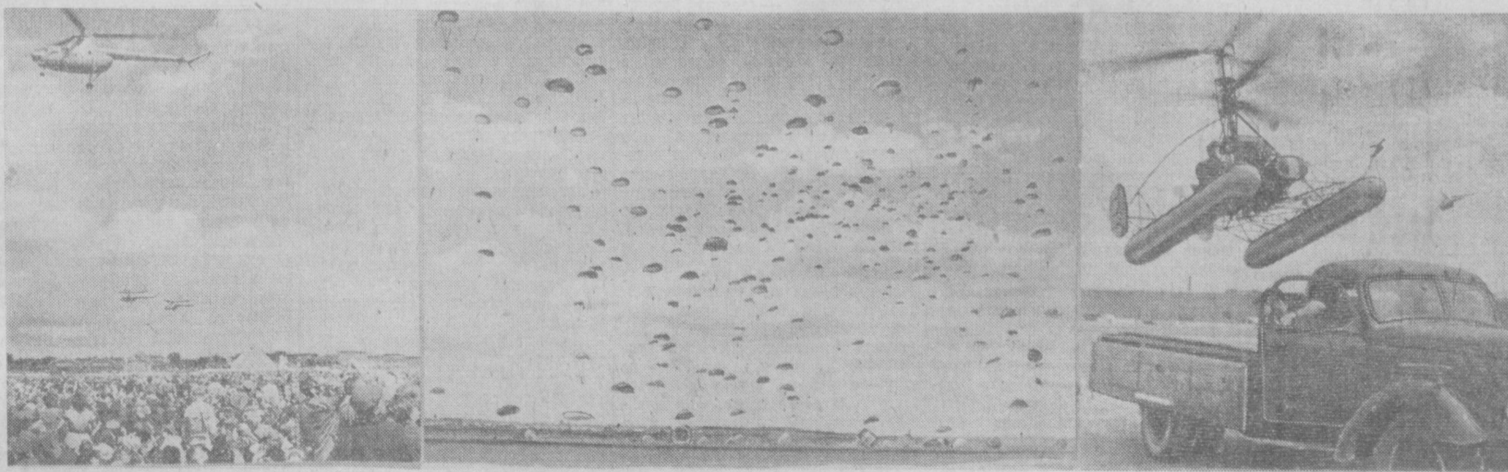
Москва, 20 июля. Авиационный праздник в честь Дня Воздушного Флота СССР на аэродроме Центрального аэродрома Союза ССР имени В. П. Чкалова в Тушине. На снимках: 1. Флагианский вертолет в полете. 2. Групповой прыжок парашютистов. 3. Взлет вертолета «К-10» с грузовой автомашиной. Фото В. Янкова, Б. Третьякова и В. Соболева. (Фотохроника ТАСС).
