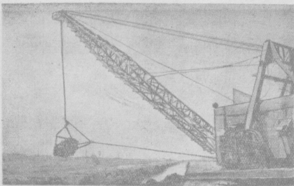
В Голодной степи ширится ирригационное строительство. Хорошо трудится на сооружении главной водной магистрали бригада шагающего экскаватора, которую возглавляет Григорий Биндус. Прокладывая русло канала по целине, его бригада вдвое перевыполнила месячное задание. На снимке: шагающий экскаватор Г. Биндуса на прокладке Голодностепского канала в районе города Янгй-Ера. Фото К. Разыкова. (Фотохроника УзТАГ).
