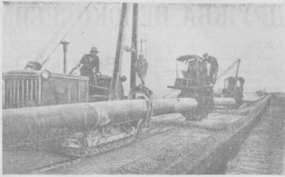
На строительстве газопровода Джаржак — Бухара — Самарканд — Ташкент. На снимке: подготовка труб и опусканию в траншею. Фото В. Сироткина.
