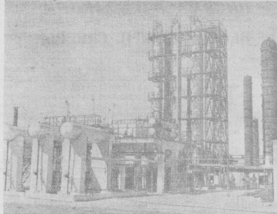
Ферганская область. На Ванновском нефтеперерабатывающем заводе пущена газофракционирующая установка. Раньше ценные газы пропали, бутан и другие продукты переработки нефти сжигались, сейчас с помощью газофракционирующей установки эти газы разделяются, и наиболее ценные фракции, как пропиленовая, бутеновая, отправляются на химические заводы, где используются как сырье для изготовления синтетического каучука, капрона, искусственного шелка, различных пластмасс и т. д. На снимке: новая газофракционирующая установка. Фото Г. Бойко. (Фотохроника УзТАГ).
