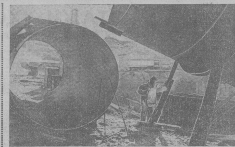
Полным ходом идет строительство Хамзинской насосной станции на трассе Аму-Бухарского машинного канала. Девять ее мощных агрегатов поднимут воду на высоту 49 метров. Фото А. Усманова. (Фотохроника УзТАТ).
