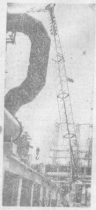
В третьем квартале этого года будет сдан подпускательные работы цех производства ацетилена на Новокимском химическом комбинате. НА СНИМКЕ: монтаж оборудования одного из цехов производства ацетилена. Фото Г. ЯСТРЕВОВА.
