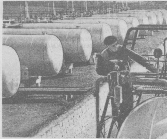
ТАТАРСКАЯ АССР. Ежедневно на промыслах республики добываются миллионы кубометров попутного нефтяного газа. Его переработка ведется на Миннибаевском газобензиновом заводе. На снимке: производственный парк, куда поступает жидкий газ с Миннибаевского завода.
