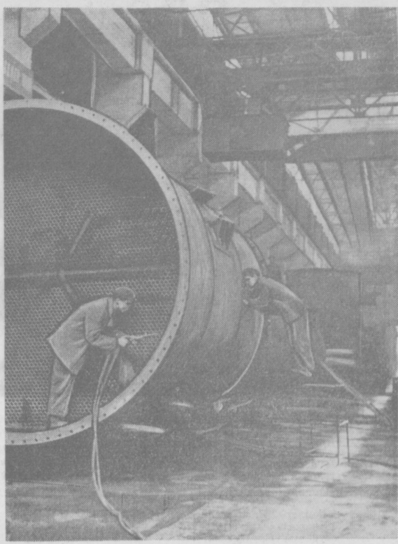
Чирчикский завод «Узбекхиммаш» начал серийный выпуск выпарных аппаратов диаметром 3.200 миллиметров для сахарной промышленности. НА СНИМКЕ: сборка выпарного аппарата.
