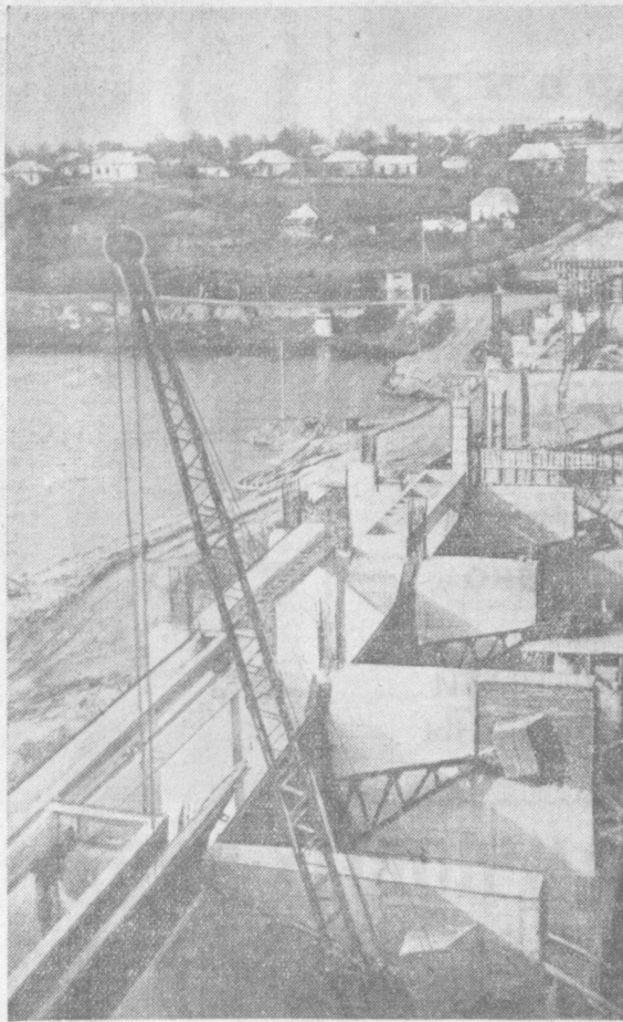
На реке Южный Буг в г. Гайворон Кировоградской области строится межрайонная гидроэлектростанция без машинного зала. На строительном объекте широко применяется сборный железобетон. В 1962 году Гайворонская ГЭС должна дать электроэнергию Гайворонскому и соседнему Уляновскому районам. Фото Г. ВЕРУШКИНА. (Фотохроника ТАСС).
