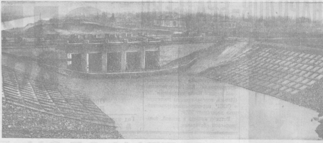
На Южном Голодностепском канале закончено строительство повторного сооружения. Его пропускная способность — 270 кубометров воды в секунду. На этом снимке вы видите сооружение перед пуском. Скоро в его котлован хлынет сырдарьинская вода. Фото А. ПАЛЕХОВА.
