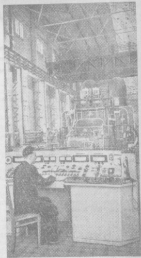
В нашей стране тепловые электростанции, работающие на природном газе, мазуте, торфе, доменных шлаках, вырабатывают примерно 80 процентов всей электроэнергии. На снимке: машинный зал Черепетской ГРЭС (Тульская область). На втором плане виден трубоагрегат мощностью 150 тысяч киловатт. (Фотохроника ТАСС).
