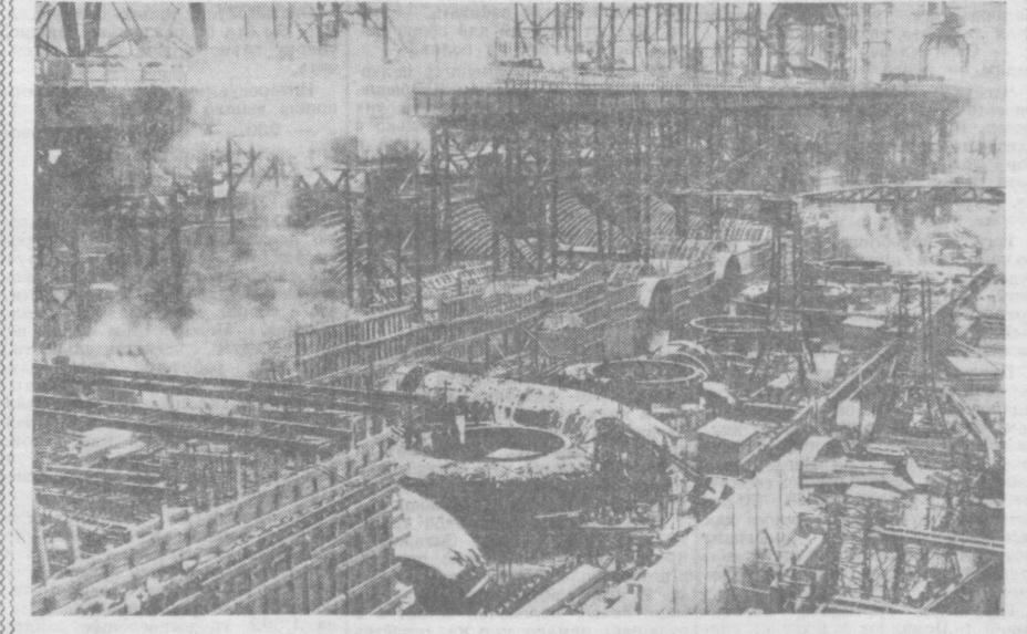
2. ОГНИ ленинской электростанции все ярче разгораются в далекой Сибири. Величественная Ангара... «Реной электричества» называют ее энергетик. На этой реке будет создан каскад электростанций. Счет уже начат. Действует Иркутская ГЭС, а ныне по течению реки широко развернулось строительство крупнейшей в мире Братской ГЭС. Ее мощность — 4.500 тыс. квт. В машинном зале ГЭС будет установлено 20 гидротурбин по 225 тысяч квт. Почти четыре Волжского в одном агрегате. Таков размер советской электростанции. НА СНИМКЕ: строительство Братской ГЭС. Фото И. Перка. (Фотохроника ТАСС).
