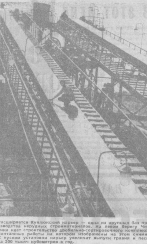
Расширяется Куйлюнский карьер — одна из крупнейших баз производства нерудных строительных материалов. На левом берегу Чирчика идет строительство дробильно-сортировочного комплекса, монтажные работы на котором изображены на этом снимке.
