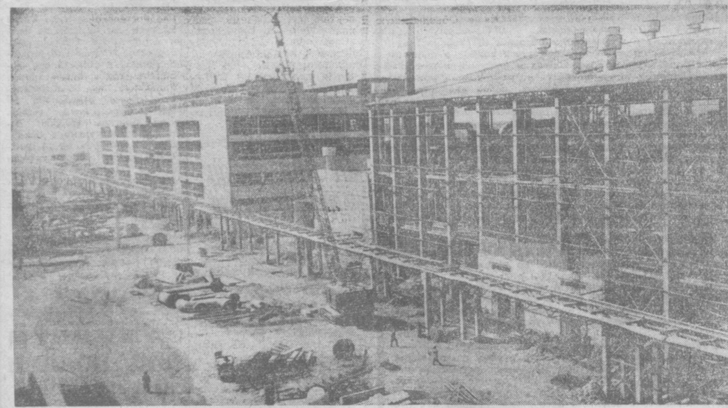
Комплекс цехов экстракции (слева) и аммофоса.
