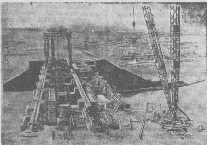
Уголок строительства плотин Фархадской ГЭС. (вид сверху). Фото С. Безнова. (Фотохроника УэТАГ).
