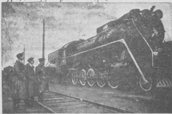
На Коломенском заводе имени Куйбышева сконструирован и построен новый тип паровоза «Победа». Новый паровоз имеет нагрузку на ось 18 тонн. Он способен развивать скорость до 80 км. Его мощность — 2200 лошадиных сил. Фото Л. Дорского. (Фотохроника ТАСС).
