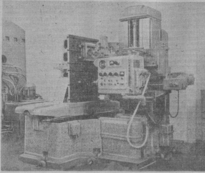
1. Ленинградский завод имени Свердлова изготовил копировально-фрезерный полуавтомат, предназначенный для обработки по копиям ковочных и вырубных штампов, металлических моделей и различных изделий, имеющих пространственно-сложную форму. Работа в станке ведется по копиям, изготовленным из дерева, алюминия, чугуна и стали в масштабе 1:1. Копирный прибор для пространственных и контурных работ действует по индуктивному способу, что обеспечивает большую плавность обвода контура. Изменение чисел оборотов шпинделя осуществляется за счет поворота трех рычагов. Для получения постоянной скорости подачи на копире в станке предусмотрен интегри-
