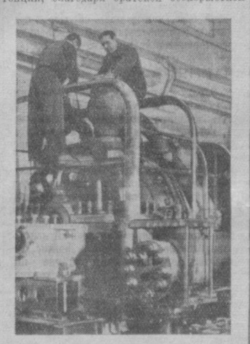
Будущий венгерский машиностроительный завод «Ланг» увеличивает выпуск локомобилей, турбин и другого промышленного оборудования. На снимке: сборка турбины, изготовляемой по заказу Польской Народной Республики.
