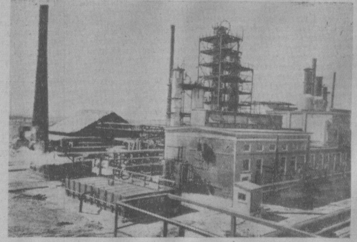
В Омске сооружается нефтеперерабатывающий завод. В конце апреля дали промышленную продукцию крекинг-установки, предназначенные для получения высокооктановых сортов бензина и керосина из мазута. Все механизмы работают хорошо. Апрельский план завод перевыполнил. На снимке: общий вид крекинг-установки. Фото В. Липовского. (Фотохроника ТАСС).
