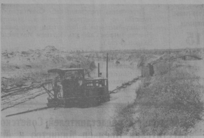
Машинно-экскаваторные станции Кара-Калыкинской АССР получили 25 малогабаритных землессосных сярдаров «ПЗУ-2», выпускаемых Ташкентским машиностроительным заводом. Они успешно используются на очистке и углублении мелкой внутриводной оросительной сети. Производительность нового земснаряда 25 кубометров грунта в час. Снаряд способен выбрасывать отсылаемый ил и песок с водой на расстояние более 50 метров. На снимке: новый земснаряд «ПЗУ-2» на углублении русла канала «Стаханов-Арна» в колхозе имени Калинин, Куйбышевского района. Фото Н. Медведева. (Фотохроника УэТАГ).
