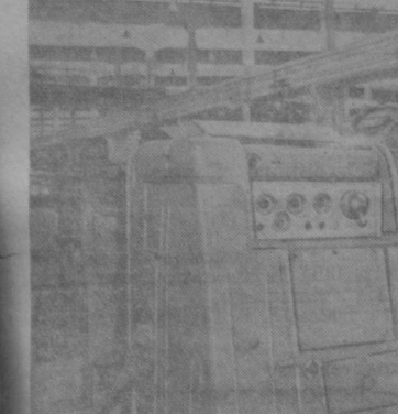
На Московском станкостроительном заводе имени Серго Орджоникидзе создан новый токарный многорезцовый гидроконтрольный станок-полуавтомат модели 17—12, предназначенный для обработки деталей типа валов различной конфигурации. Станок работает в четыре хода без смены обрабатываемой детали. Последняя операция — чистовая обработка — производится при автоматическом включении двойной скорости, после чего станок автоматически выключается. На снимке: станок модели 17—12. Фото Н. Ситникова. (Фотохроника ТАСС).
