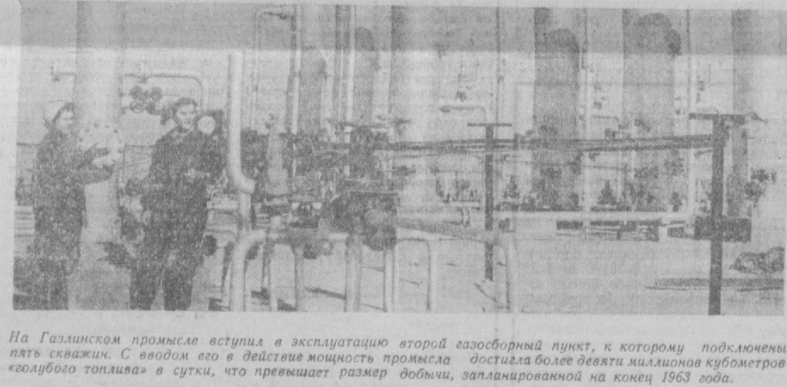
На Газликинском промысле вступила в эксплуатацию вторая газосборный пункт, к которому подключены пять скважин. С вводом его в действие мощность промысла достигла более девяти миллионов кубометров «голубого топлива» в сутки, что превышает размер добычи, запланированной на конец 1963 года.
