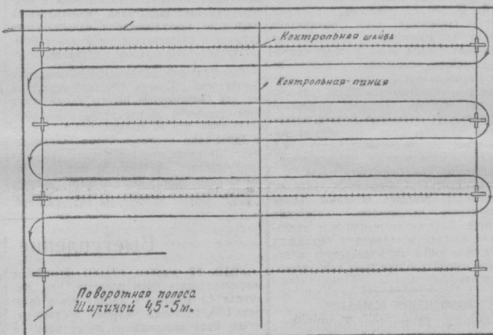
Рис. 2. Схема движения агрегата и установки мерной проволоки.
